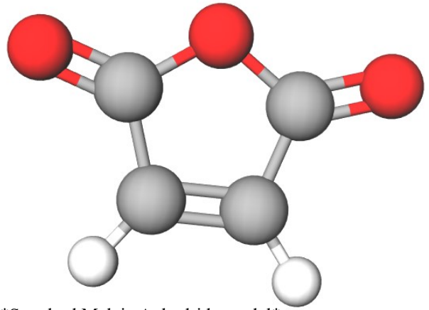
*Standard Maleic Anhydride model*
